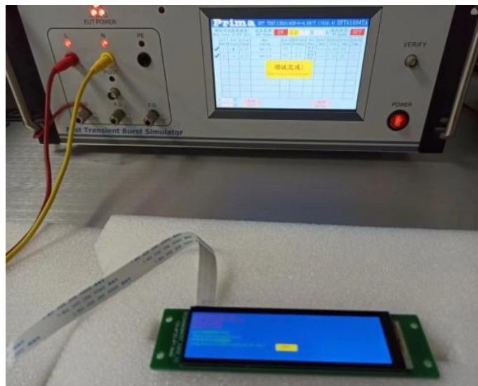
图 3-4 群脉冲测试图
